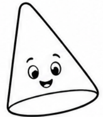
Oblique cone
