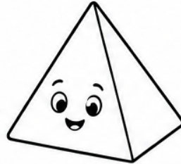
Pyramid
