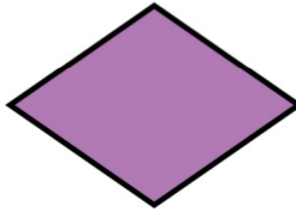
Rhombus
